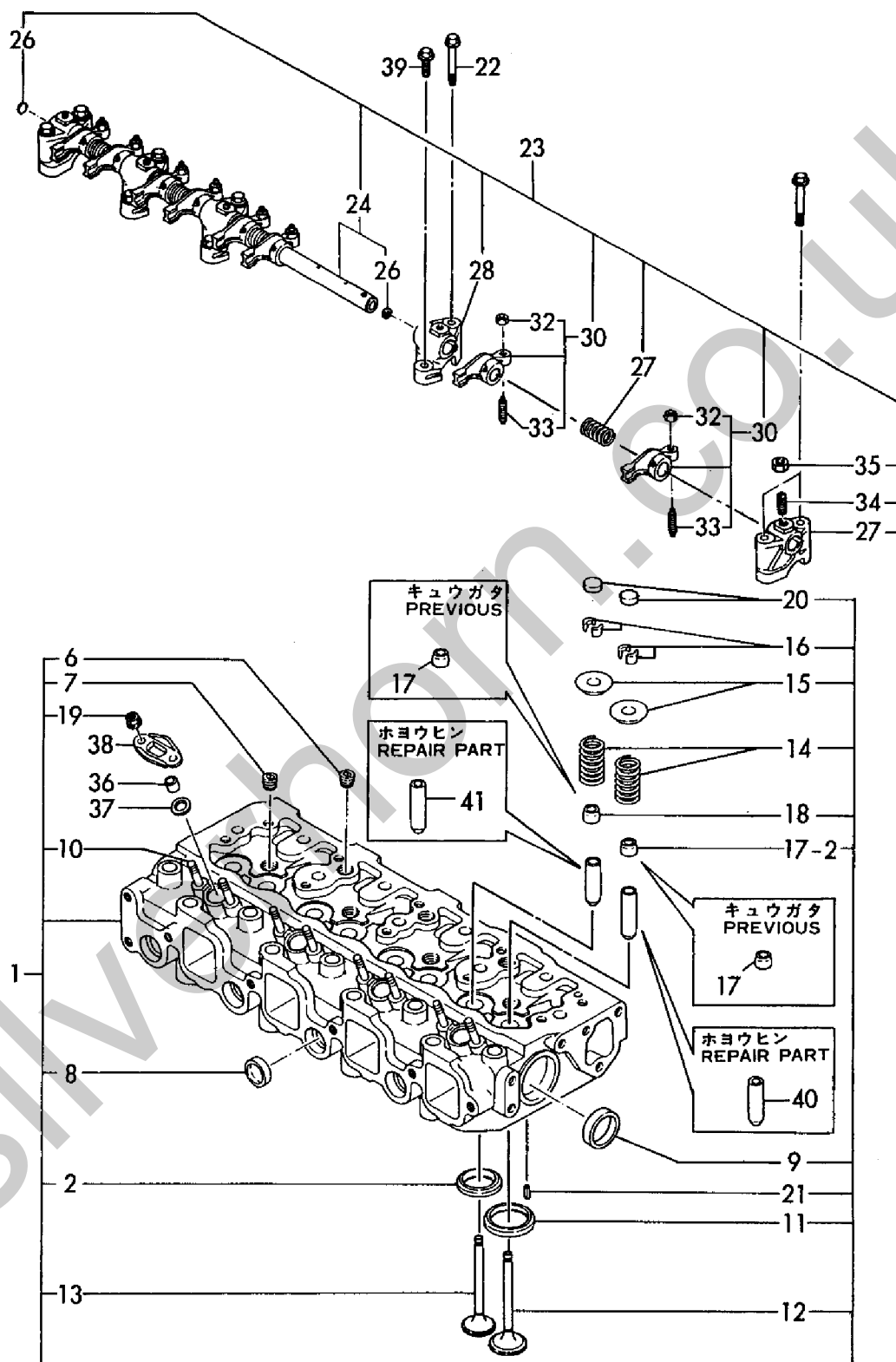
Fig. 9 シリンダヘッド CYLINDER HEAD
