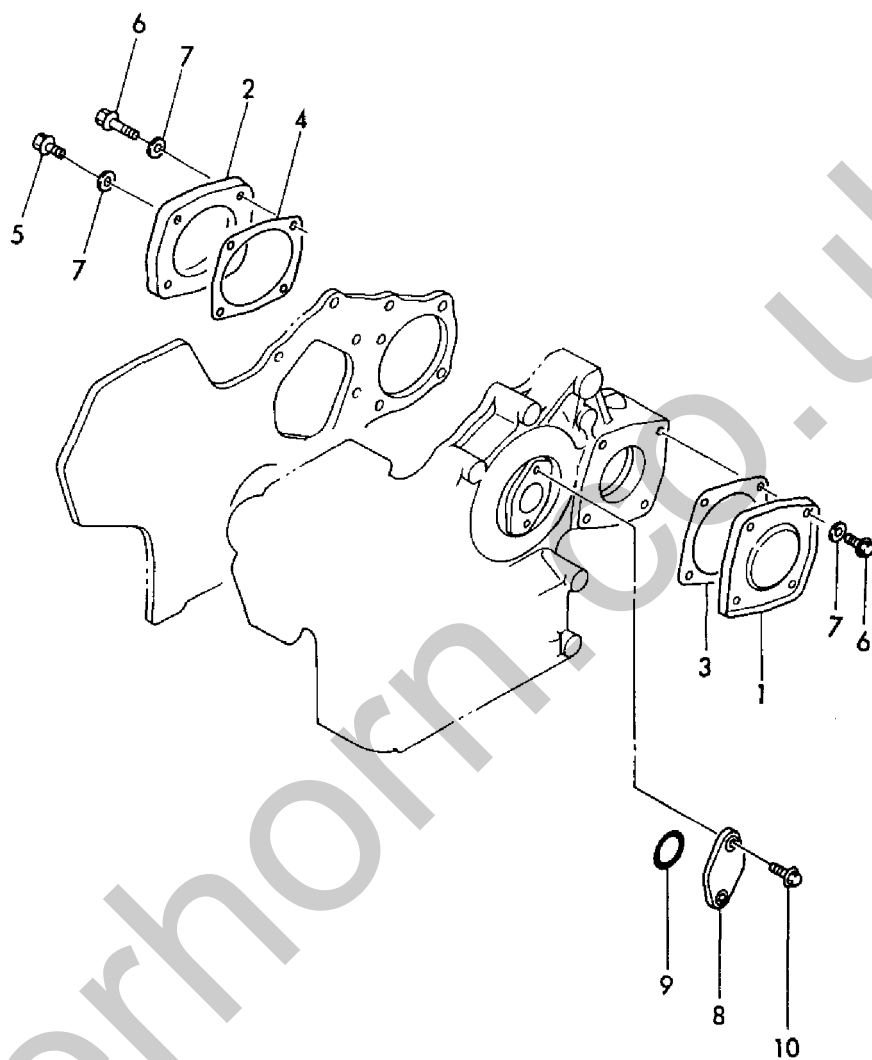
Fig. 6 H0ポンプ フタ HYD. OIL PUMP COVER
