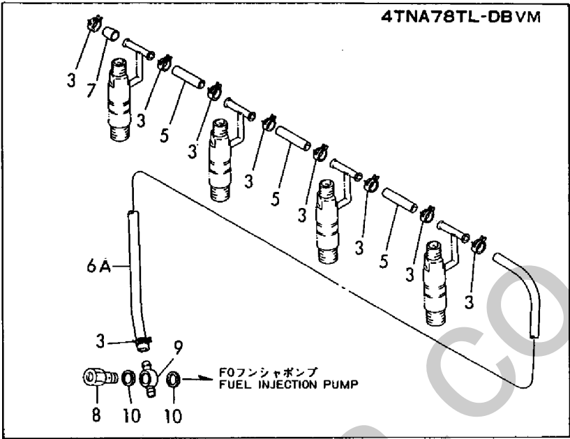
FOモドシパイプ FUEL RETURN LINE
