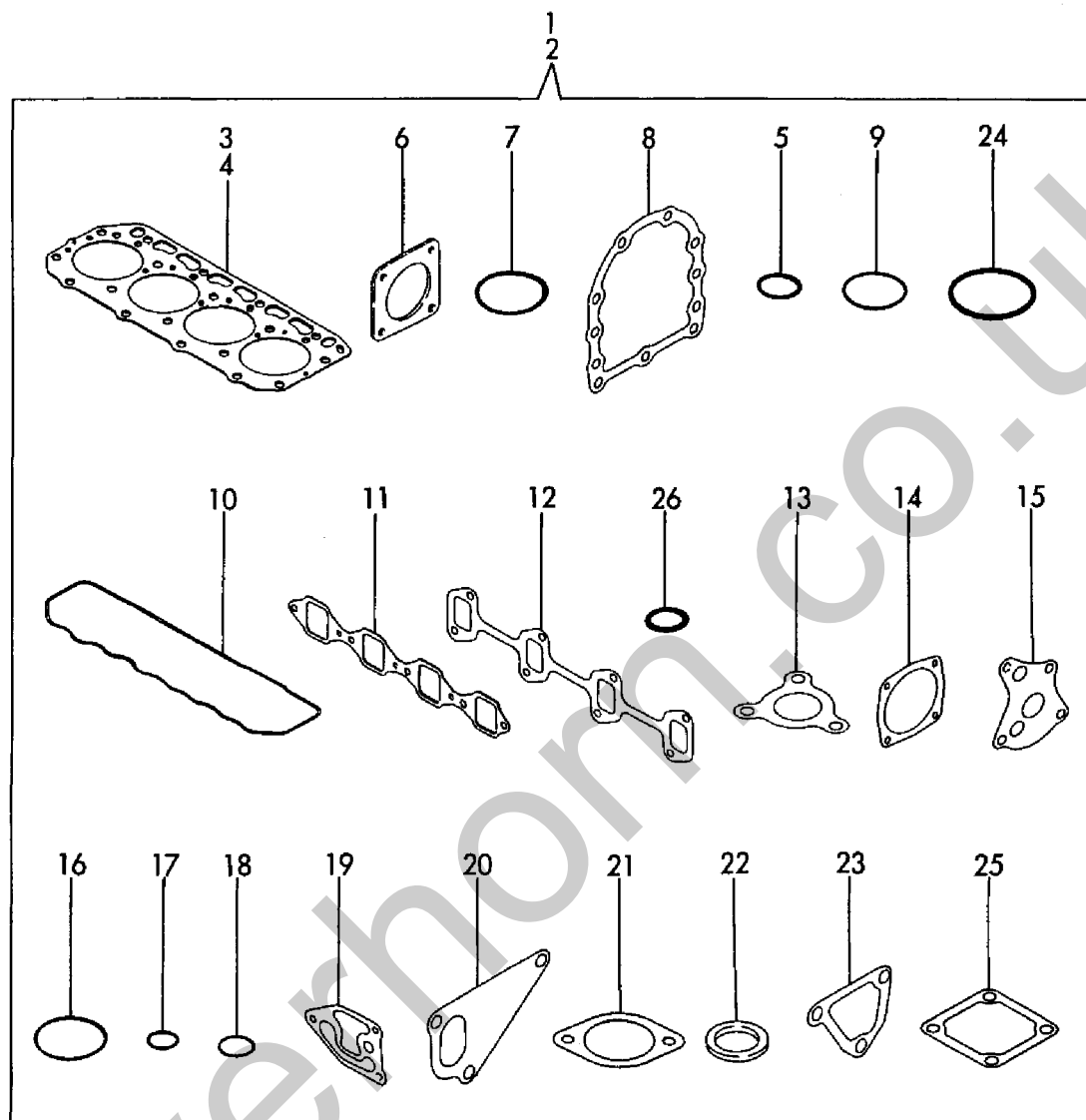
Fig. 45 パッキンセット(オプション)&コウグ GASKET SET (OPTIONAL) & TOOL
