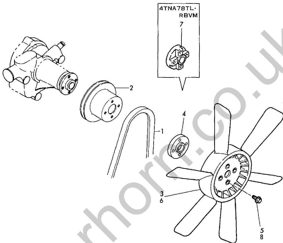
Fig. 29 CWファン& ファンプーリ
