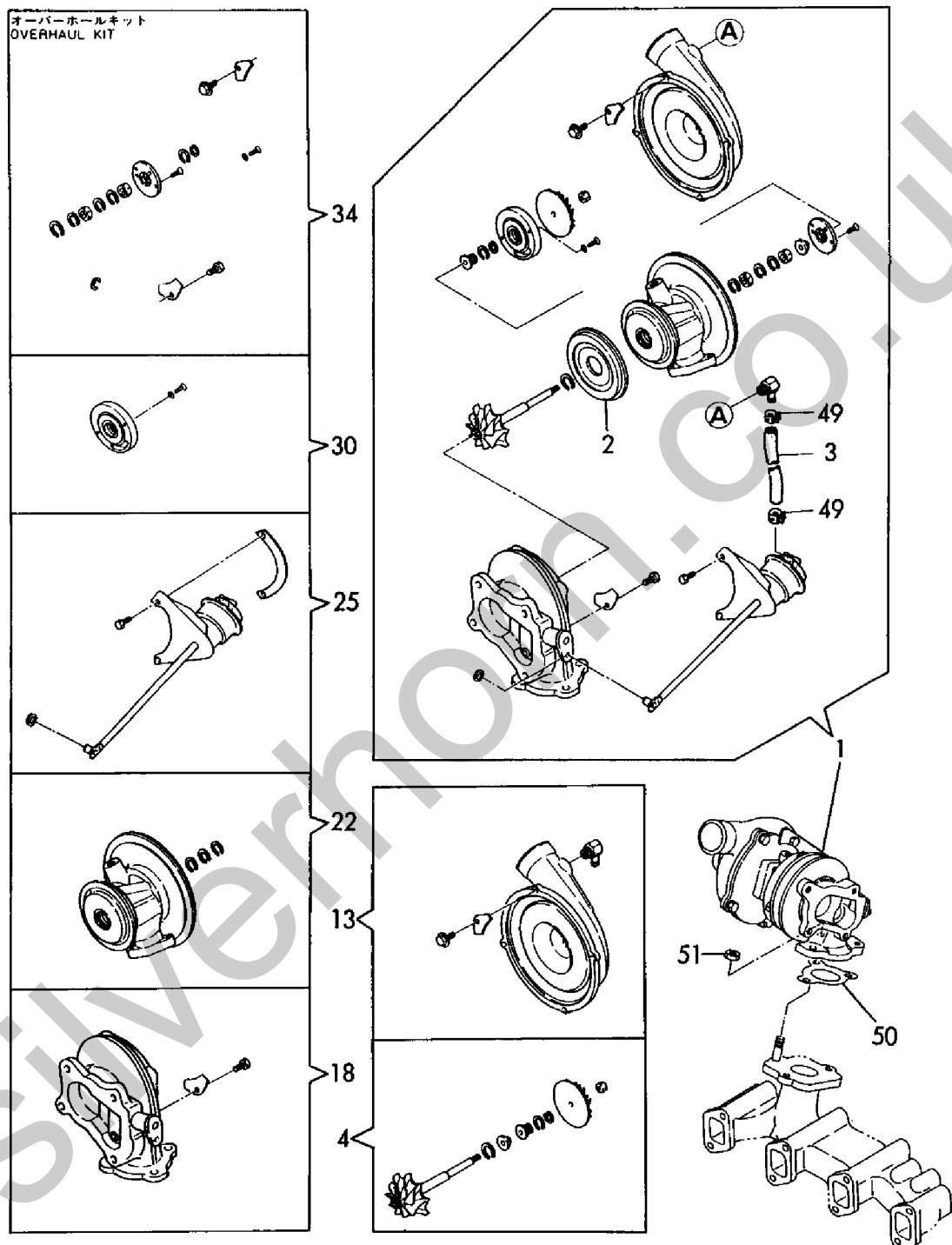
Fig. 13 タービン TURBOCHARGER
