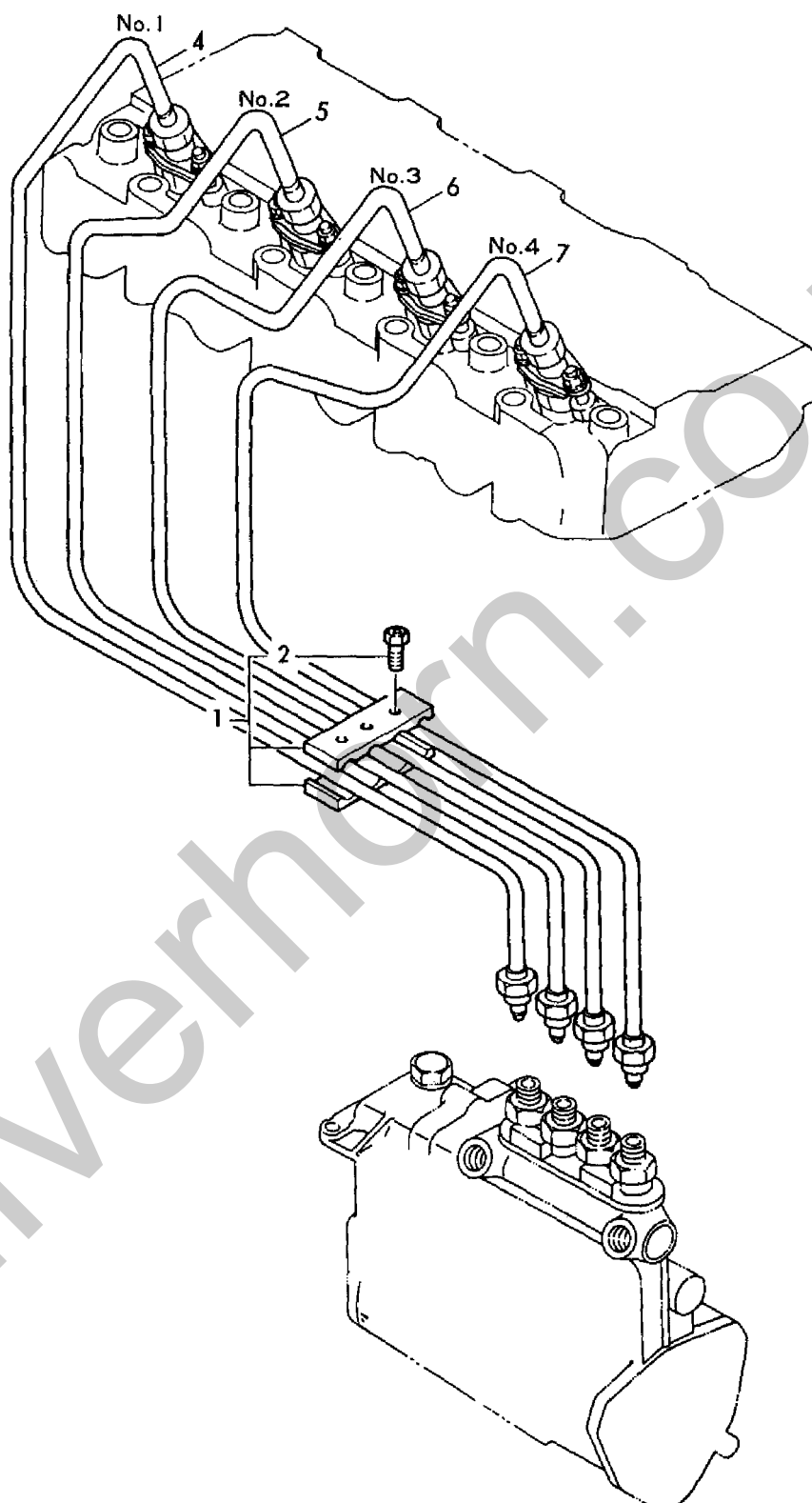
Fig. 36 FOファンシャパイプ FUEL INJECTION LINE
