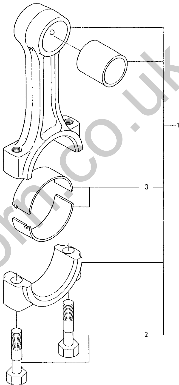
Fig. 17 コネクティングロッド CONNECTING ROD
