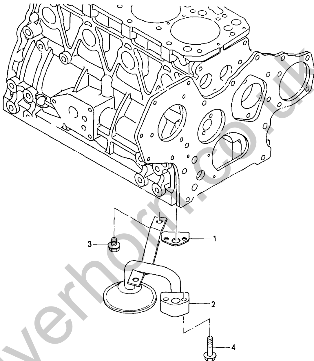
Fig. 23 LOキューニューカン LUB. OIL SUCTION PIPE
