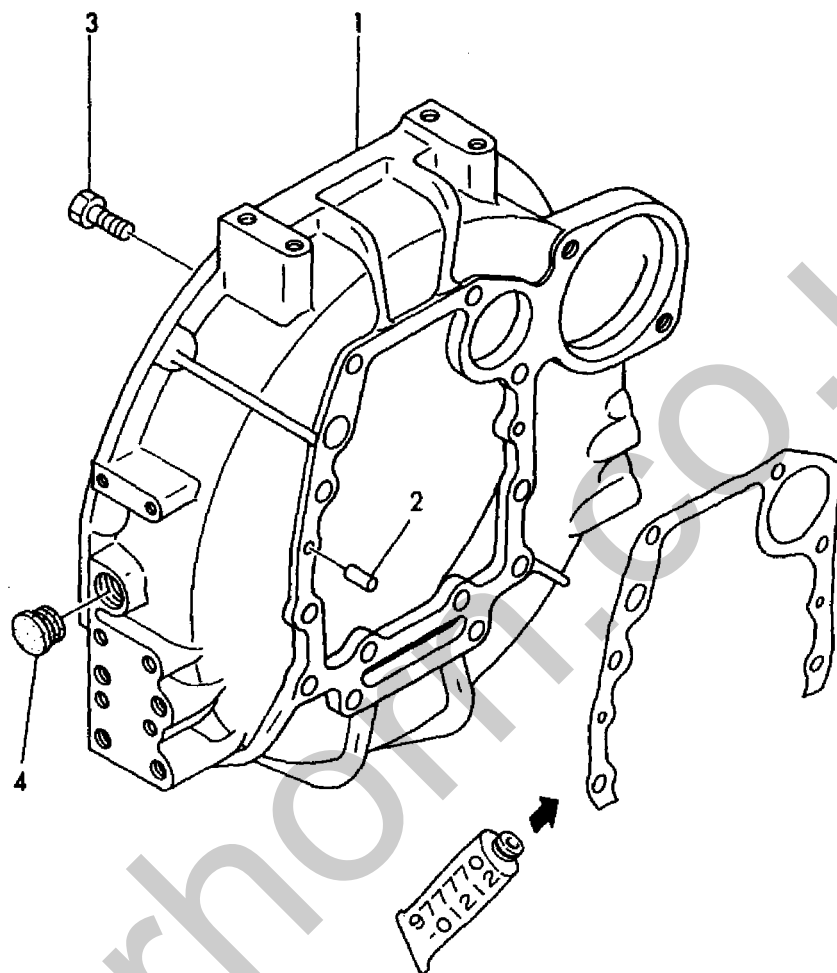
Fig. 3 フライホイールハウジング FLYWHEEL HOUSING
